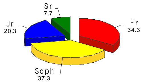
GATs *
