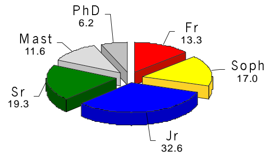
GATs *
